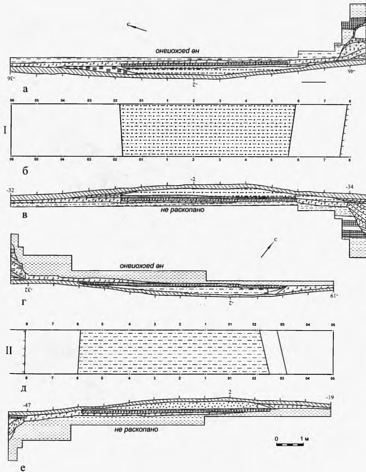
Рис. 20. Второе Троицкое городище. Остатки стен в траншеях II (I) и III (II). Планы (б, д) и профили бортов: а — западного, в — восточного, г — юго-восточного, е — северо-западного.
