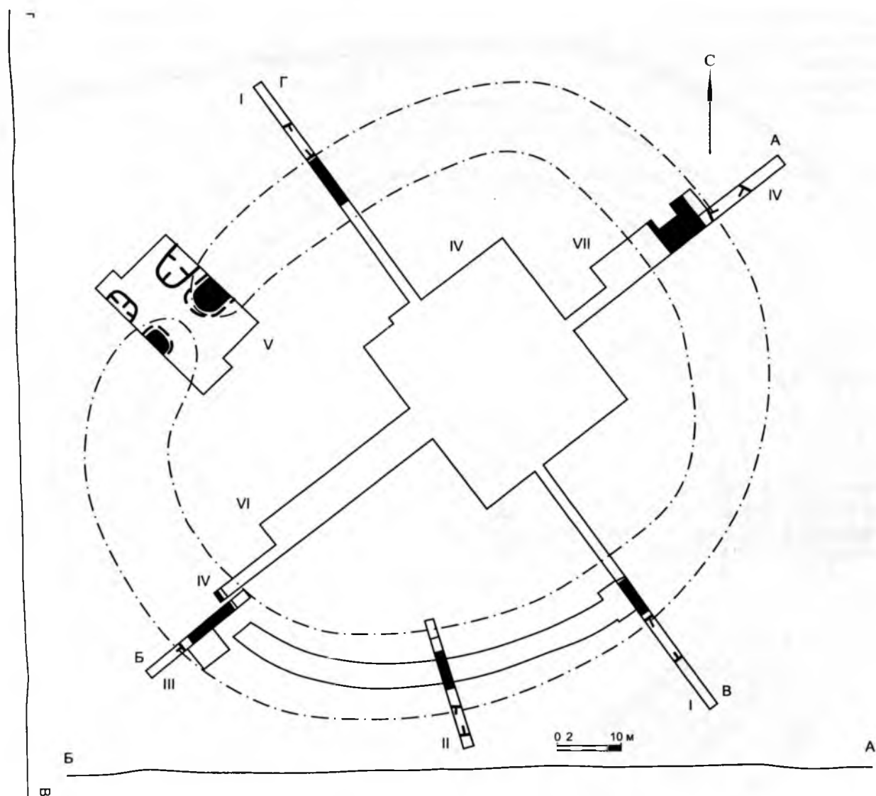
Рис. 7. Второе Троицкое городище. План, разрезы и расположение раскопанных участков: траншей I–IV и раскопов IV–VII. Штрих-пунктир – граница распаханых стен, заливка черным – первичное тело стен, линии с бергштрихом – верхние границы рвов.
