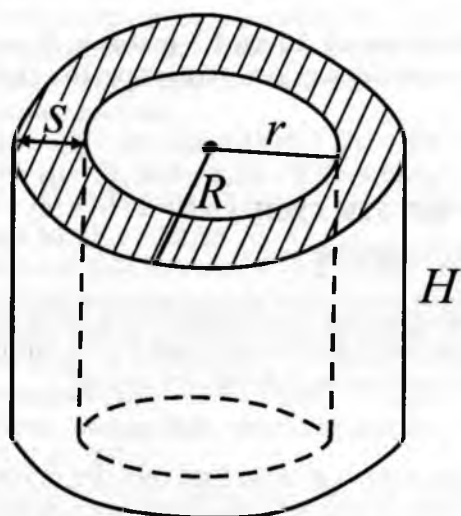
Рис. 48. Схема вычисления объема цилиндрического кольца, образуемого при вращении фигуры KDMB относительно центра.
