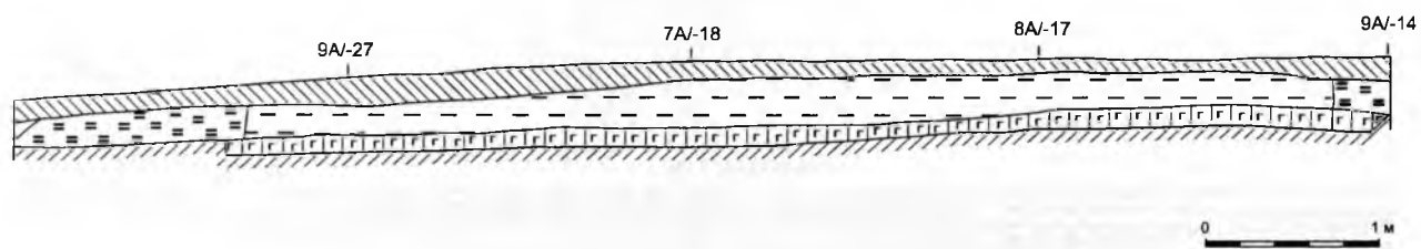
Рис. 21. Второе Троицкое городище. Северо-восточный профиль раскопа V. Деталь.
