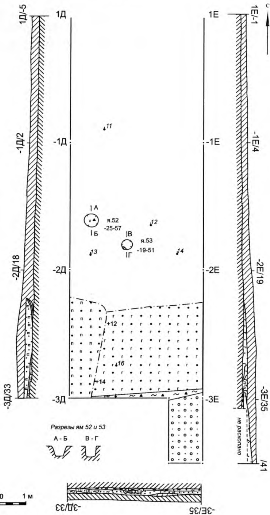
Рис. 45. Знаменское городище. Траншея VI. План и профили.
