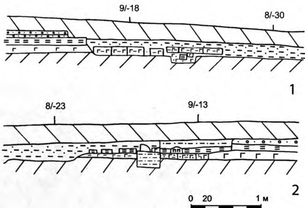
Рис. 34. Знаменское городище. Детали южного (1) и северного (2) профилей траншеи I: остатки кирпичной кладки с внешней стороны стены.
