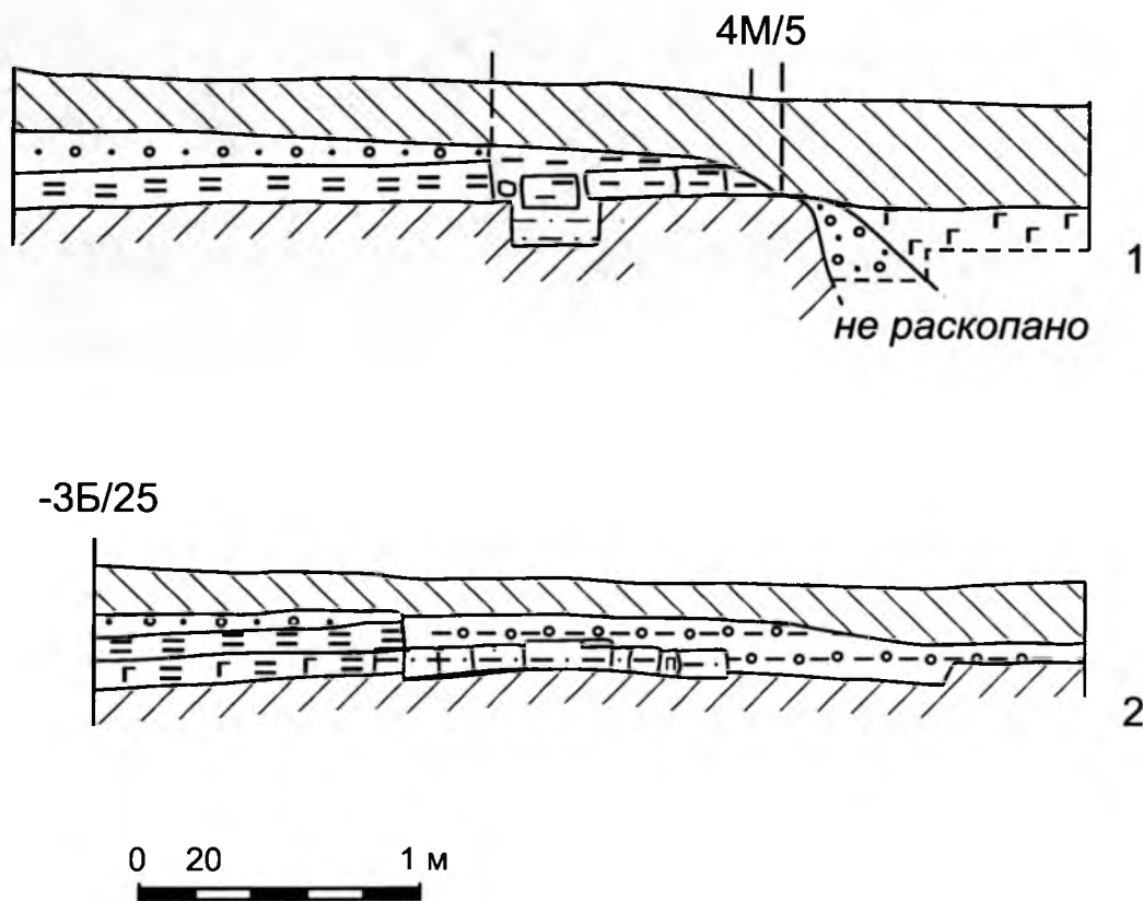
Рис. 35. Знаменское городище. Остатки кирпичной кладки. Детали профилей: северного в траншее V (1) и восточного в траншее IV (2).
