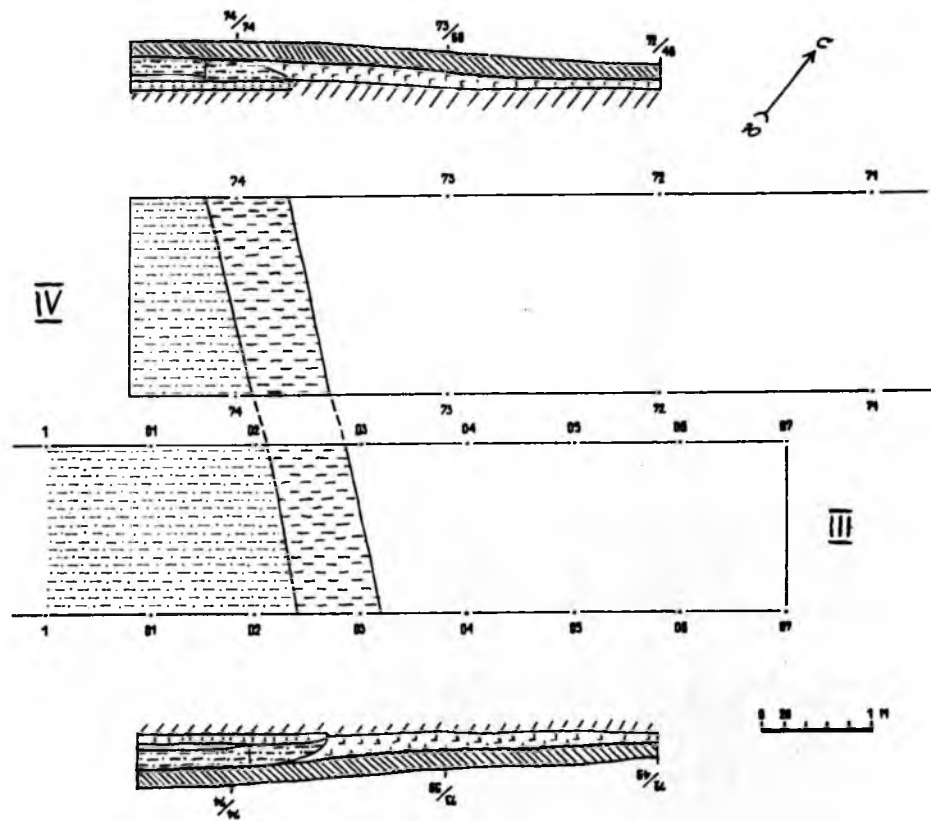
Рис. 14. Второе Троицкое городище. План схождения траншей III и IV. Профили траншей IV.
