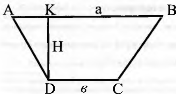
Рис. 46. Геометрическая схема сечения рва.
