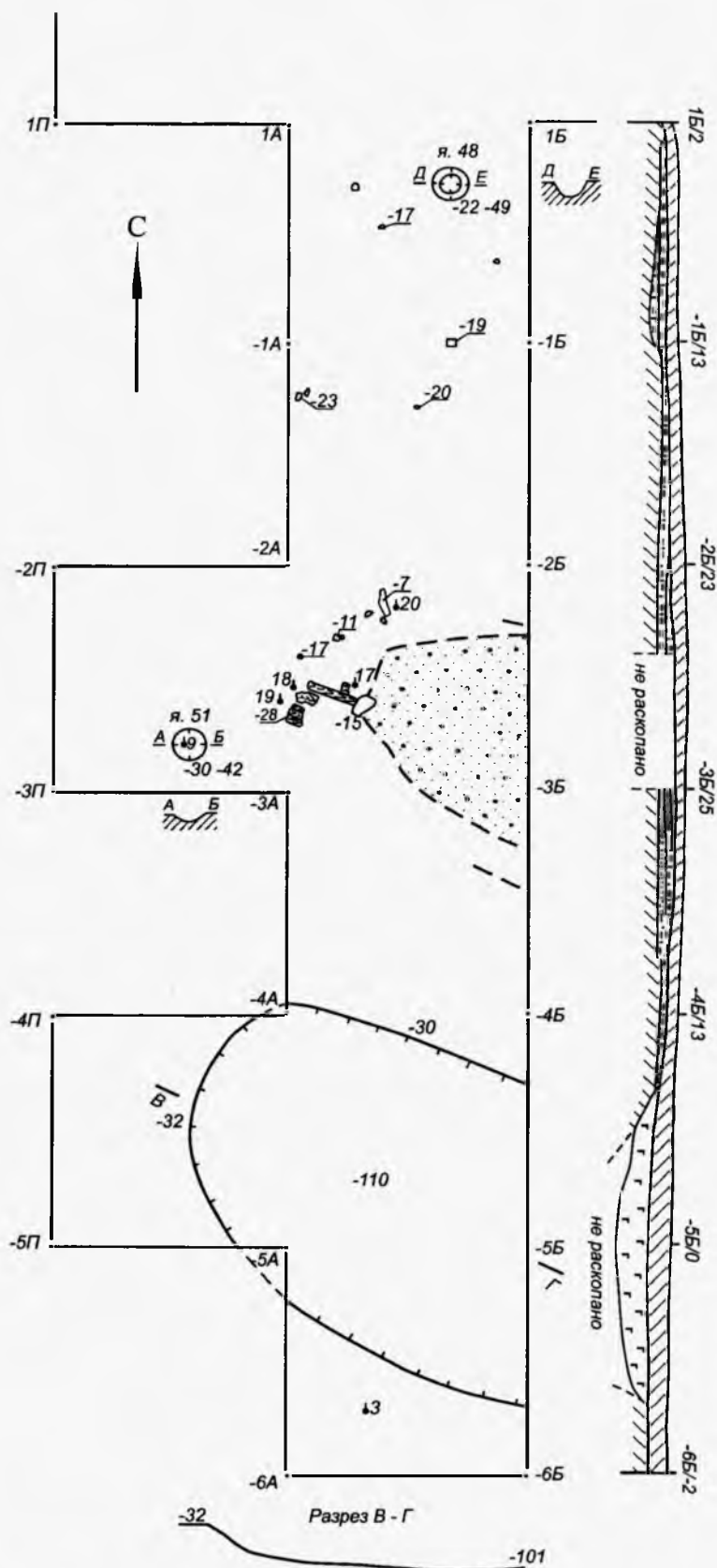
Рис. 11. Знаменское городище. План и профиль траншеи IV. Восточная сторона юго-западного входного проема. Контуры стены обозначены пунктиром.
