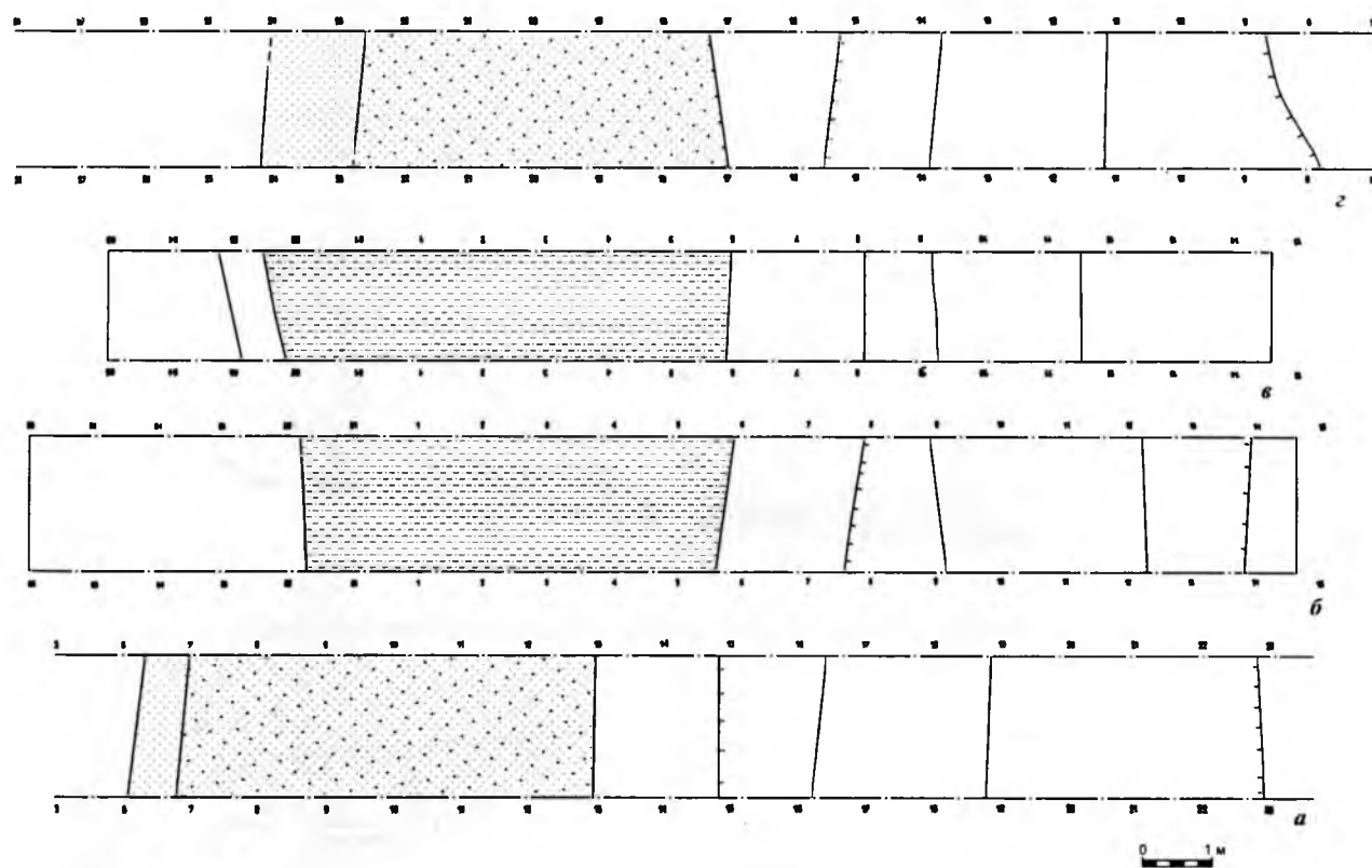
Рис. 13. Второе Троицкое городище. Глинобитные тела стен, прилегающие внутренние «пандусы» и внешние рвы. Планы траншей южной и восточной оконечностей: а – I (меж реперами 5–23), б – II (реперы 06–01, 1–15), в – III (реперы 05–01, 1–15), г – IV (реперы 7–28).
