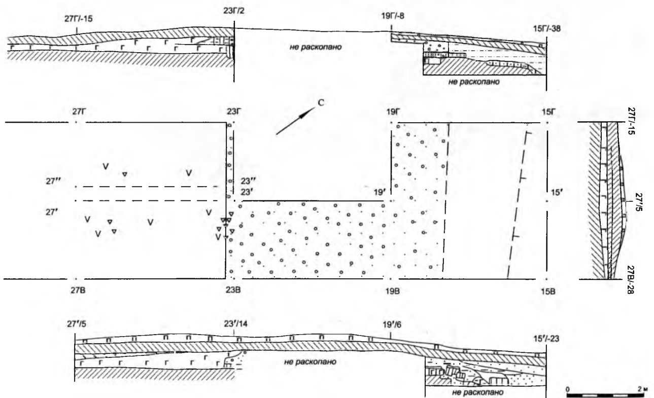
Рис. 15. Второе Троицкое городище. План и профили раскопа VII.
