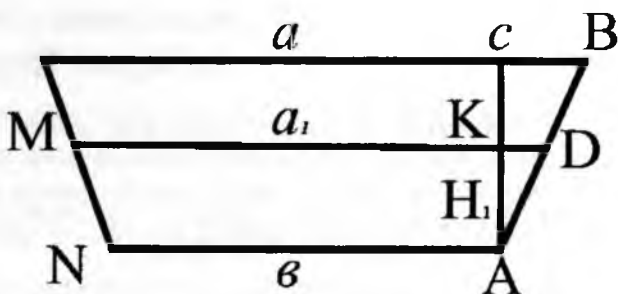
Рис. 49. Схема расчета объема развала стены во рву.
