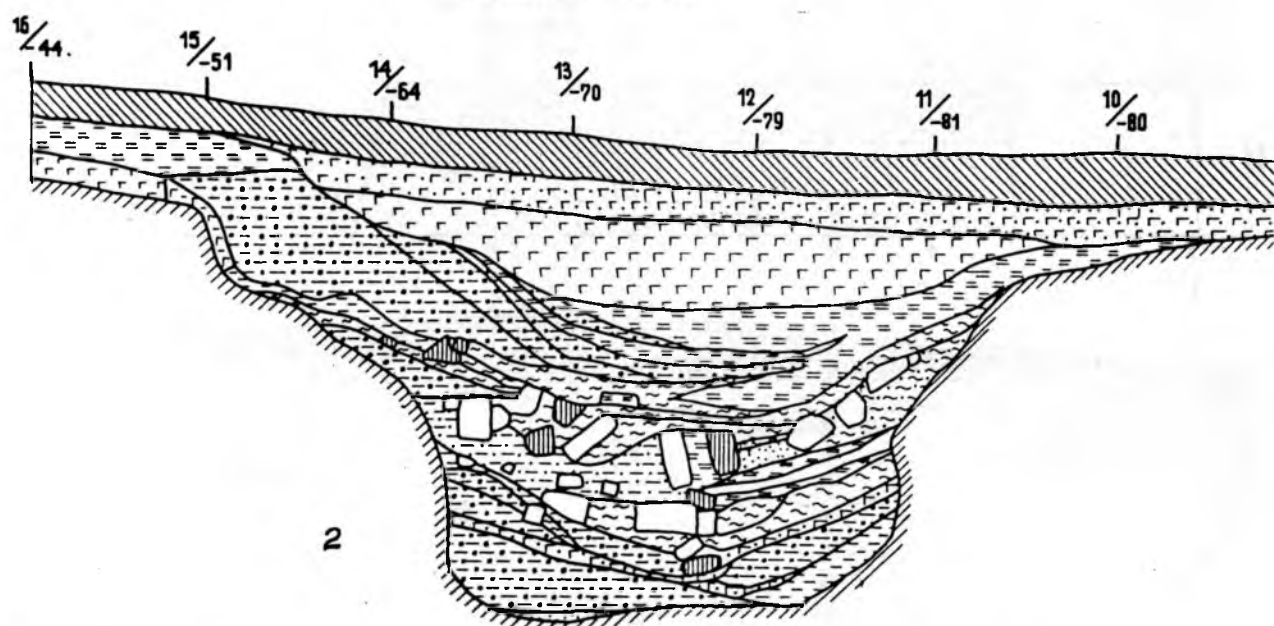
Рис. 22. Второе Троицкое городище. Траншея IV. Юго-восточный (1) и северо-западный (2) профили рва.
